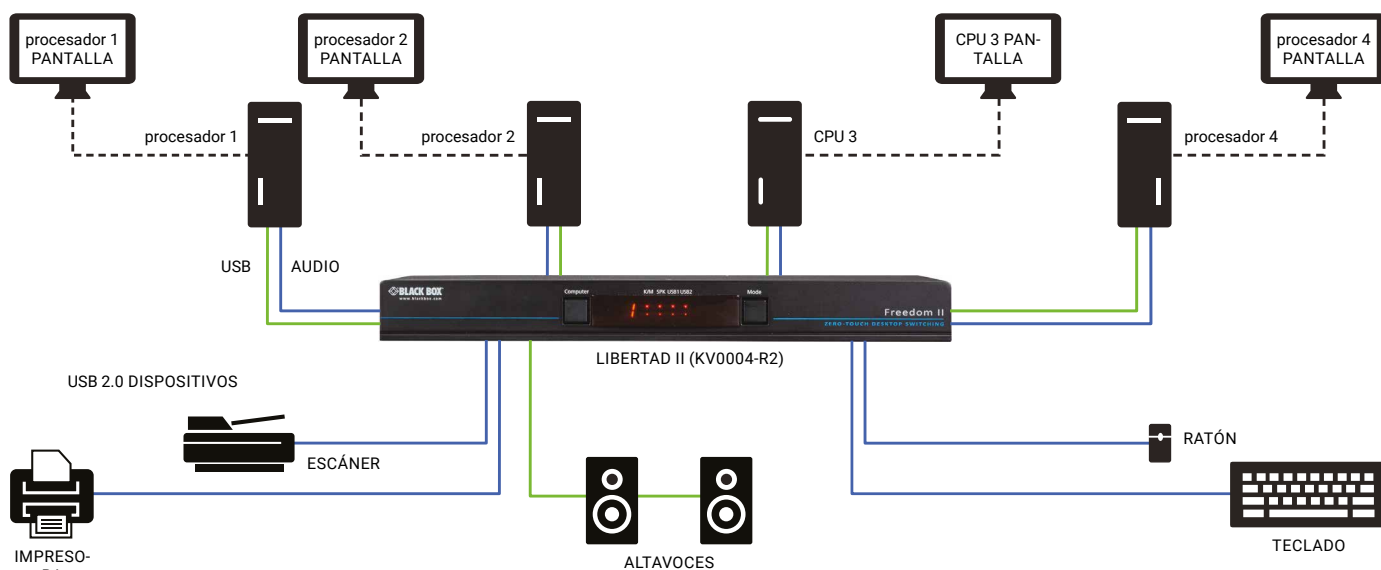
Configuración de 4 puertos Freedom II que incluye dispositivos USB 2.0
