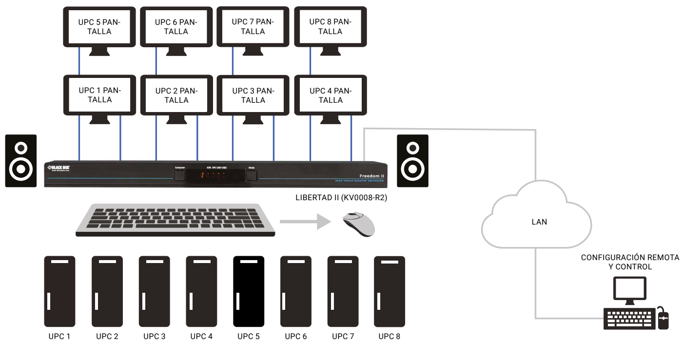
Configuración de 8 puertos Freedom II
